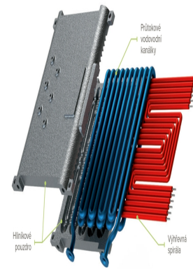
* Ilustrační 3D obrázek vyhřevné spirály s hliníkovým blokem Long Life Technology
